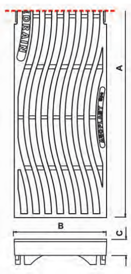
PE-HD rešetka, A15 kN
