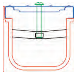
Pritrjevanje z ročico in vijakom za vroče cinkane ali inox rešetke. 1 set na kanaletu
