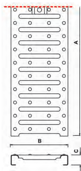
Vroče cinkana ali inox štancana rešetka z regami, A15 kN
