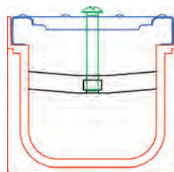
Pritrjevanje z ročico in vijakom za vroče cinkane ali inox rešetke. 1 set na kanaletu AbarWDK110
