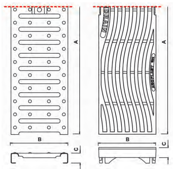
Vroče cinkana ali inox štancana rešetka z regami Awd110AZ Awd110AX
